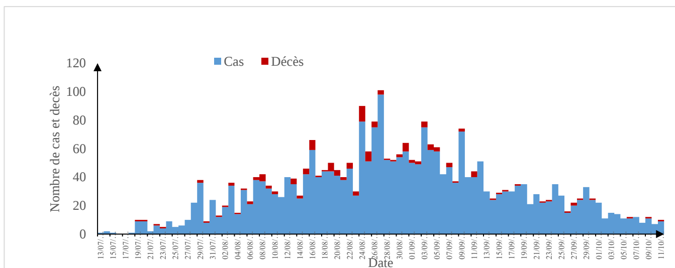
Figure 2 : Courbe journalière des cas et des décès de choléra (N=2727)
