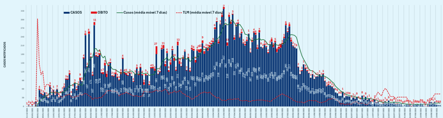
Gráfico 1: Casos e óbitos diários por data do início dos sintomas (31 de Dezembro de 2024 até 21 de Agosto 2025)
