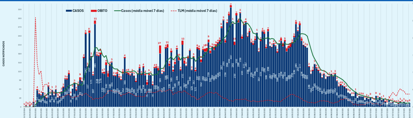
Gráfico 1: Casos e óbitos diários por data do início dos sintomas (31 de Dezembro de 2024 até 27 de Julho 2025)
