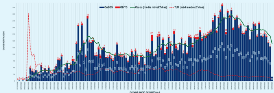
Gráfico 1: Casos e óbitos diários por data do início dos sintomas (31 de Dezembro de 2024 até 18 de Maio 2025)
